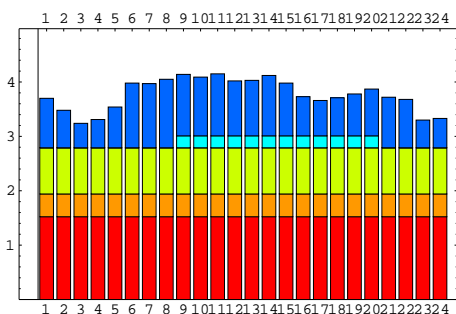
Denný priebeh dodávok a jej zloženie podľa jednotlivých dodávateľov
