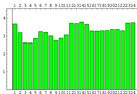
Denný priebeh plánovanej spotreby (zelený graf) a skutočných dodávok (zelený graf so žltým navýšením)
