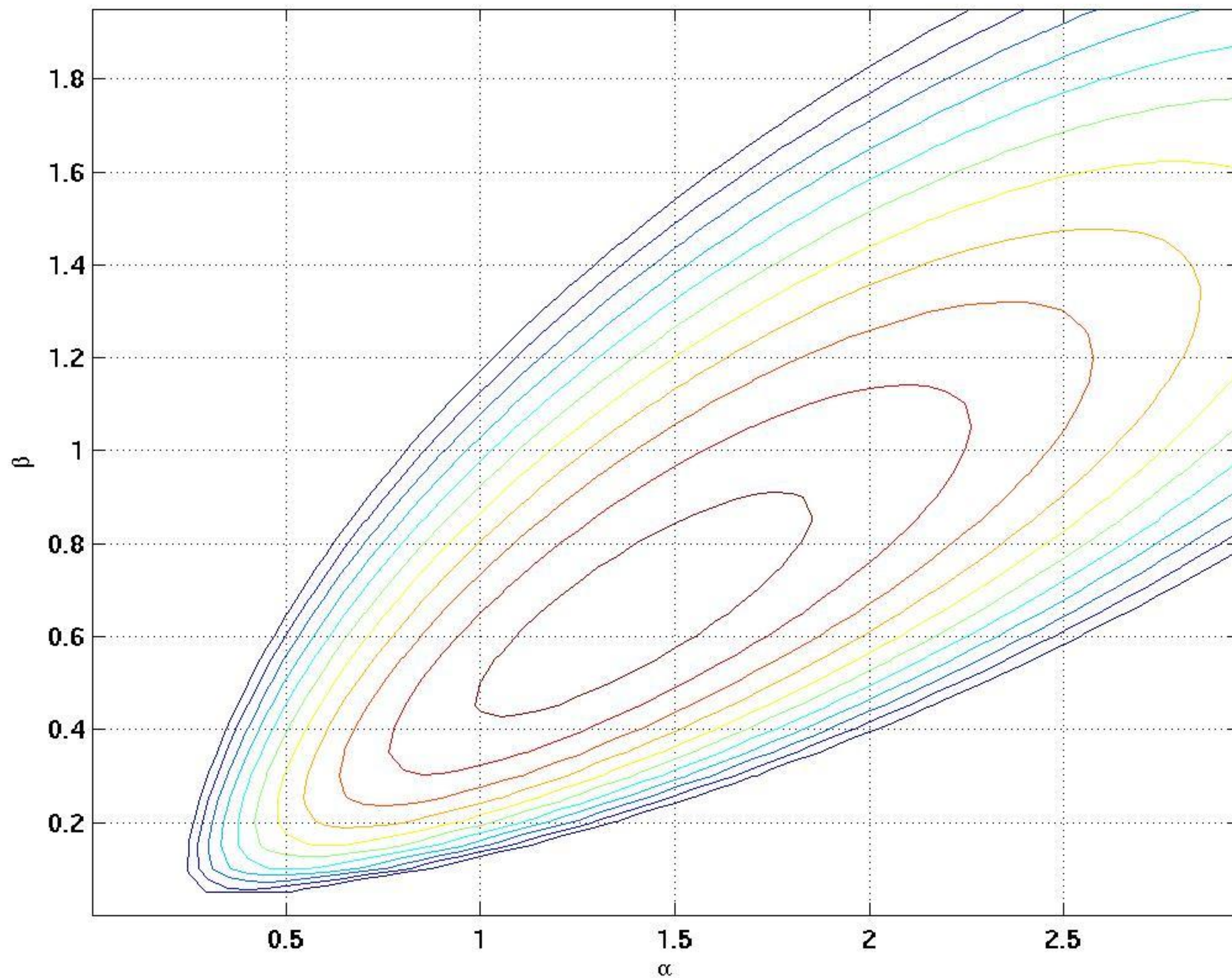
Vrstevnice funkcie \log L(\alpha, \beta)
